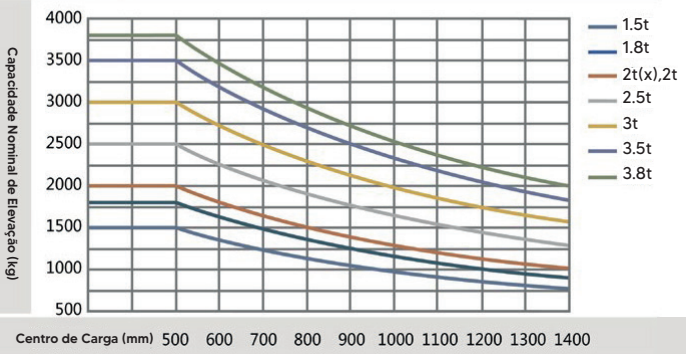
Diagrama de curva de carga
